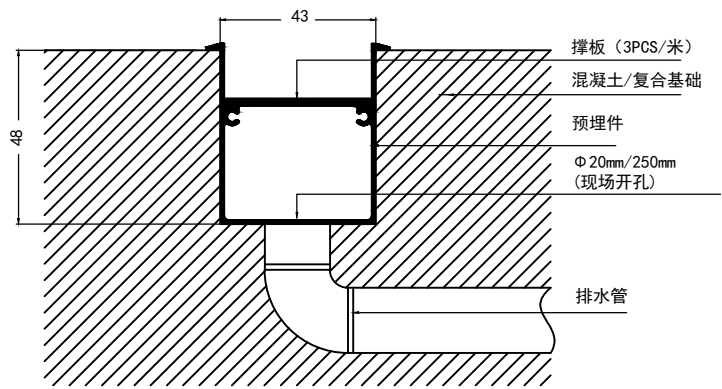
排水管系统上预埋件的安装
