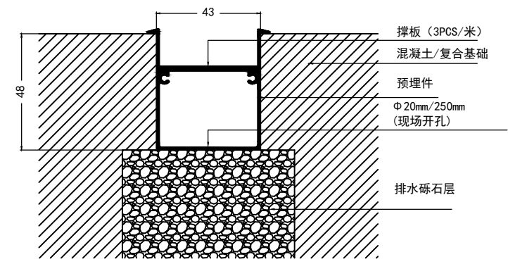
排水层上预埋件的安装
