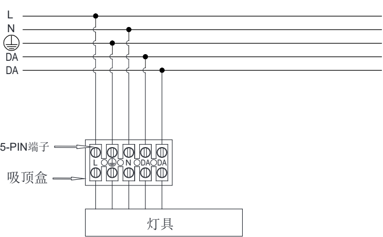
DALI调光功能
